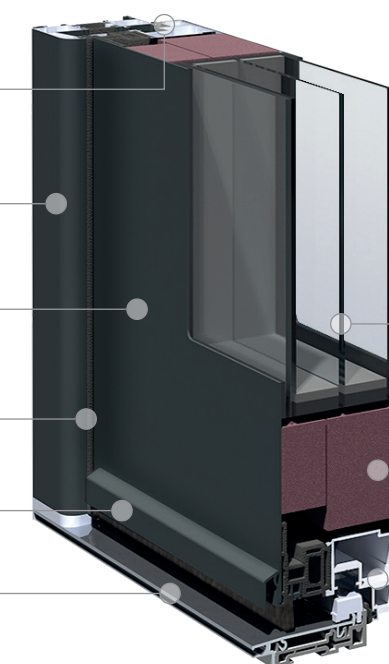
Paumelles 3D pour un réglage simplifié
