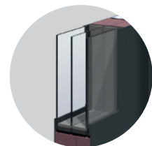
TRIPLE VITRAGE Avec une face feuilletée 33/2 en standard (44/2 ou SP10 en option) retardateur d'effraction
