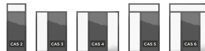
Tierces et impostes fixes
